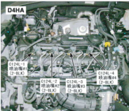
172. 发动机顶部
