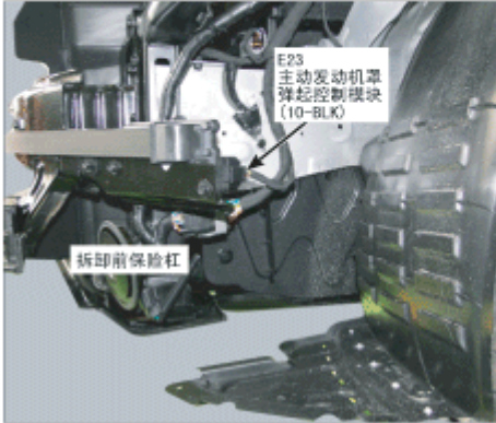
169. 前端模块左侧
